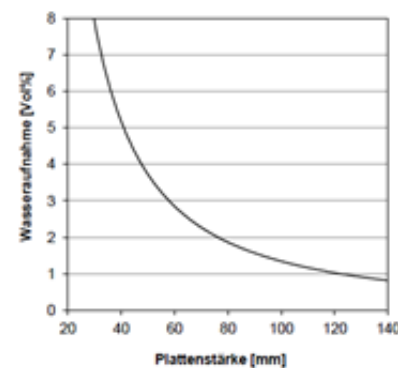
Abb. 3: Einfluss der Plattenstärke auf die Wasseraufnahme durch Diffusion (EN 12088) (Verschweißung >95 %; 30 kg/m 3 )
